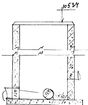
Чертеж колодца М 1:25
