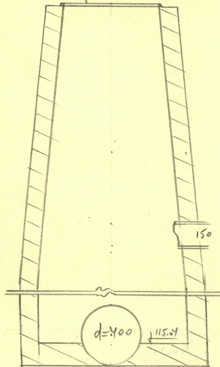
Чертеж колодца
