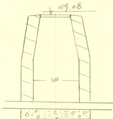
Чертеж колодца М 1:50
