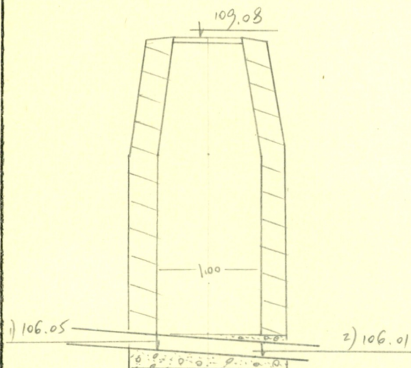
Чертеж колодца М 1:50
