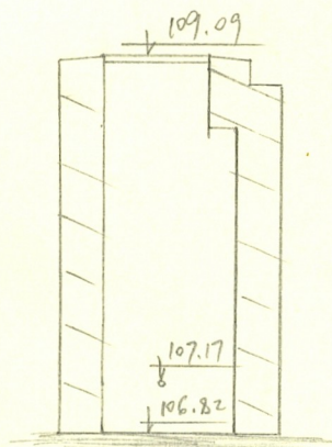
Чертеж колодца М. 1:50
