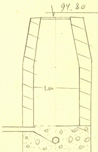
Чертеж колодца М 1:50
