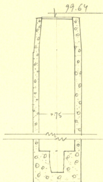
Чертеж колодца М 1:50
