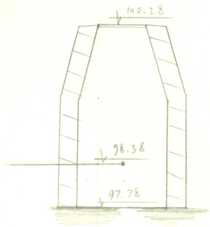
Чертеж колодца М. 1:5
