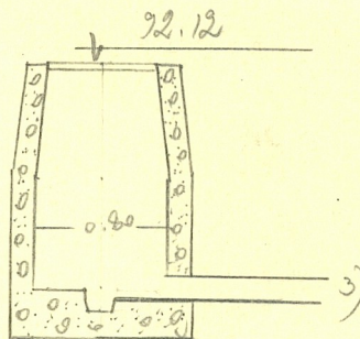
Чертеж колодца М 1:50
