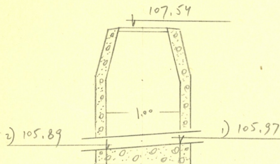
Чертеж колодца М 1:50
