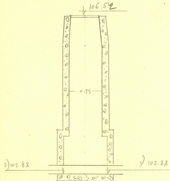
Чертеж колодца М 1:50
