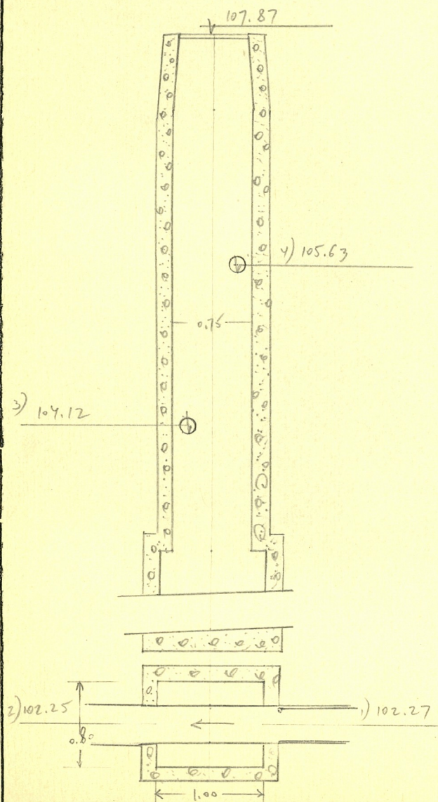
Чертеж колодца М 1:50
