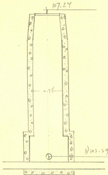
Чертеж колодца М 1:50
