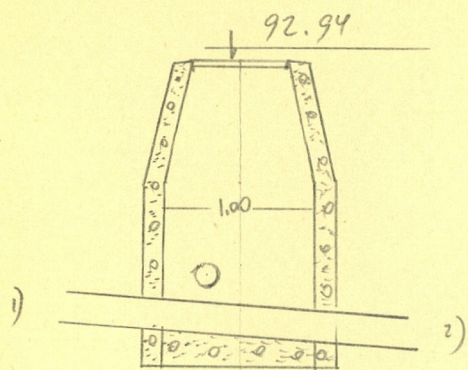
Чертеж колодца М 1:50
