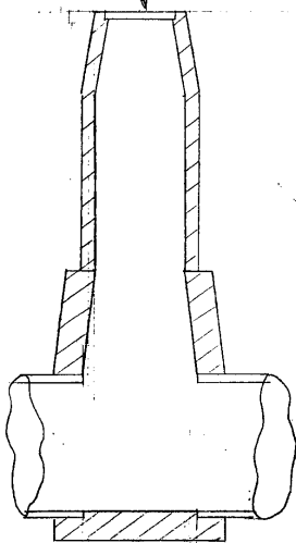
Чертеж колодца М 1:50 по А-А
