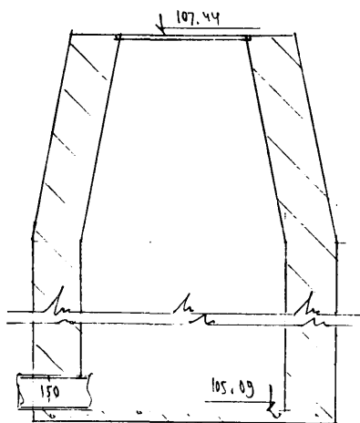
Чертеж колодца М 1:2,5
