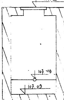
Чертеж колодца М 1:50
