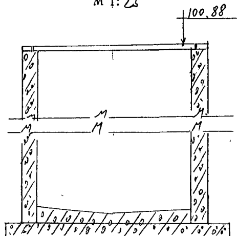
Чертеж колодца М 1:25
