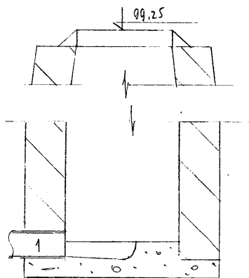
Чертеж колодца М 1:25
