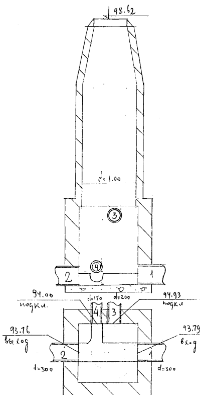
Чертеж колодца М 1:50
