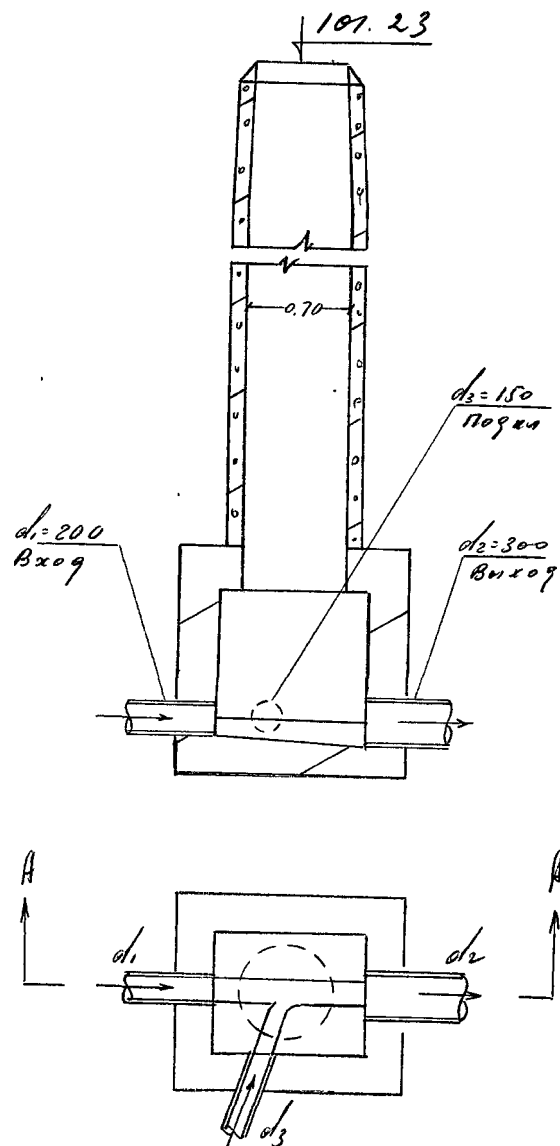
Чертеж колодца М 1:50
