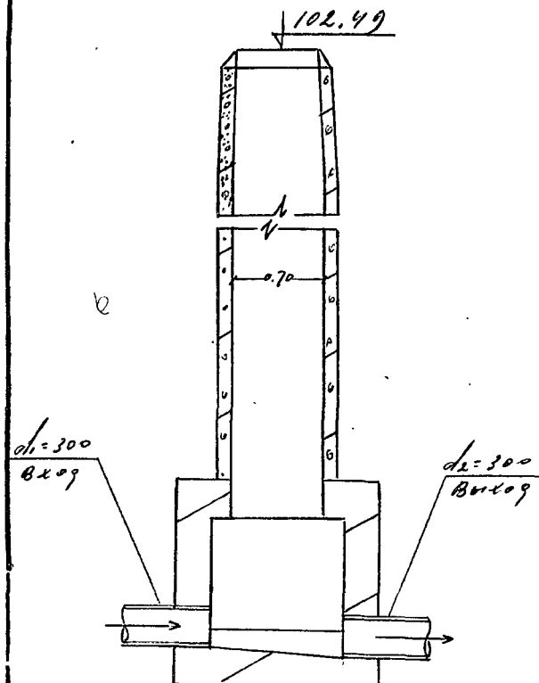
Чертеж колодца М 1:50
