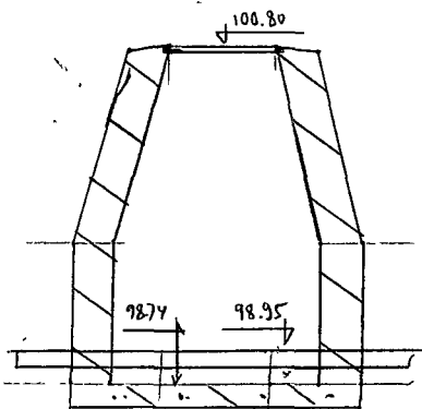
Чертеж колодца М. 1:50
