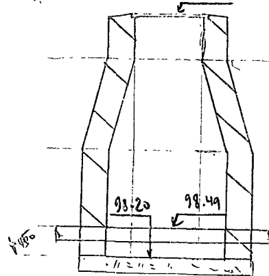
Чертеж колодца
