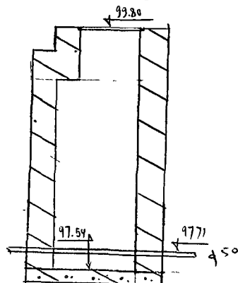
Чертеж колодца М. 1:50
