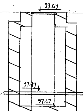
Чертеж колодца М. 1: 50
