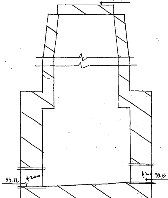
Чертеж колодца М 1:25
