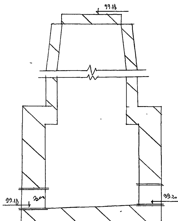
Чертеж колодца М 1:25
