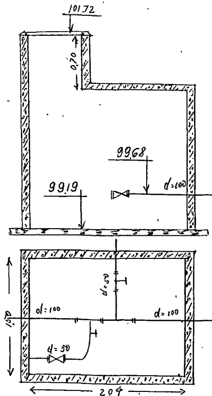
Чертеж колодца М. 1:50
