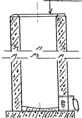
Чертеж колодца М 1:25
