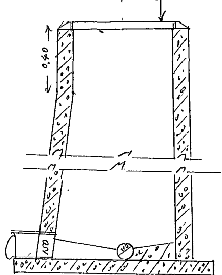
Чертеж колодца М 1: 10186
