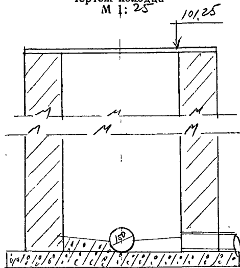
Чертеж колодца М 1:25
