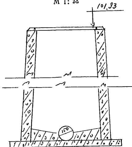
Чертеж колодца М 1:25
