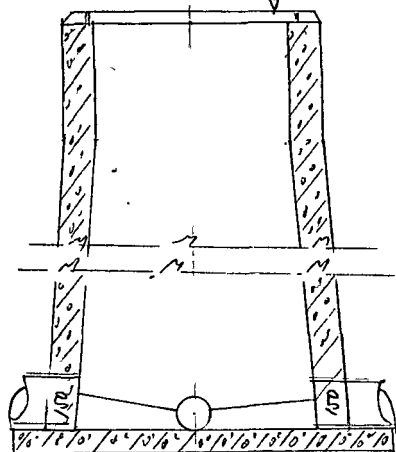
Чертеж колодца 101.94 М 1:25
