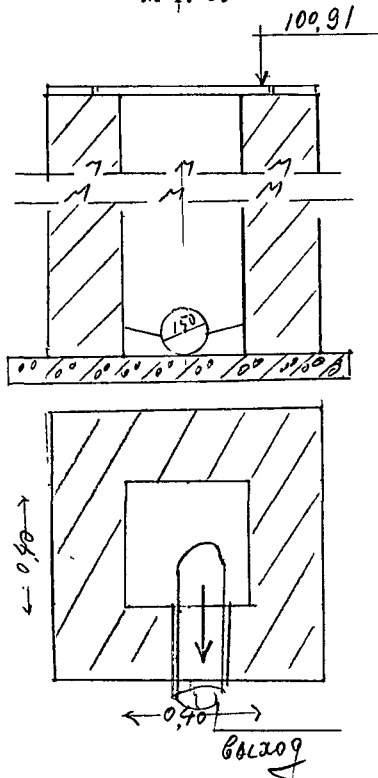
Чертеж колодца М 1:25
