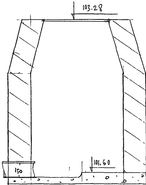
Чертеж колодца М 1:25 по А-А
