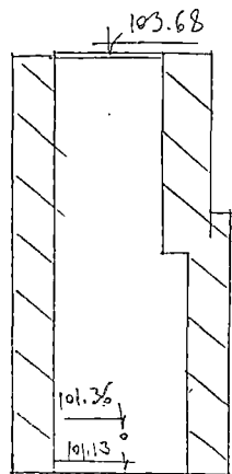
Чертеж колодца М. 1:50
