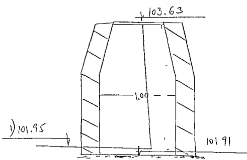
Чертеж колодца М. 1:50
