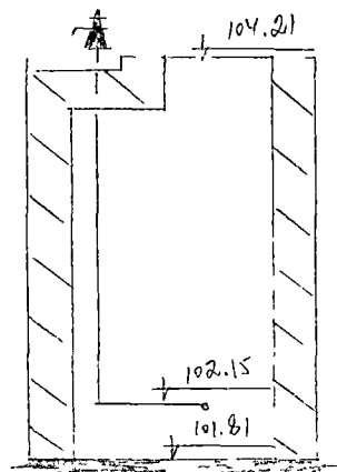
Чертеж колодца М. 1:50
