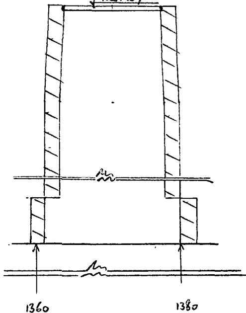
Чертеж колодца
