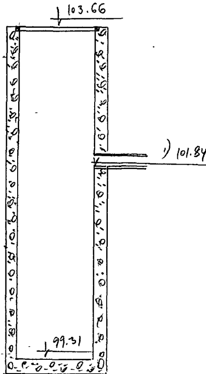
Чертеж колодца М 1:50
