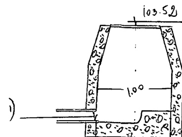
Чертеж колодца М 1:50
