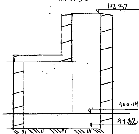
Чертеж колодца М. 1:50
