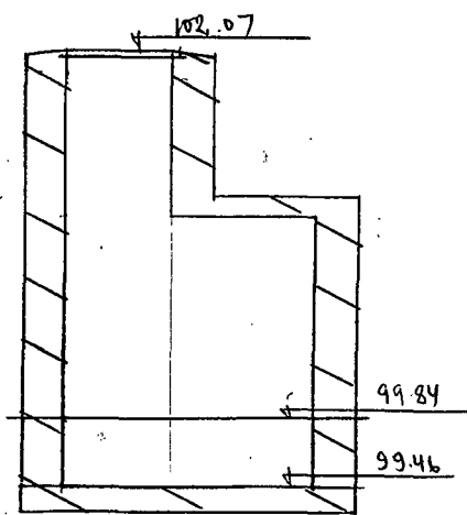
Чертеж колодца М. 1:50
