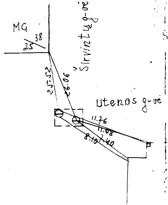
Pririšimo brėžinys:
