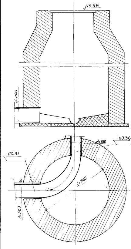
Чертеж колодца М 1:25
