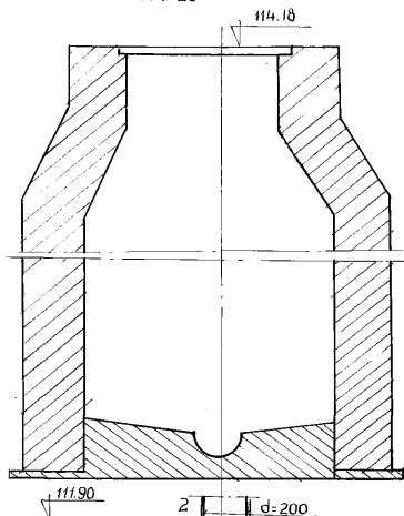
Чертеж колодца М. 1: 25
