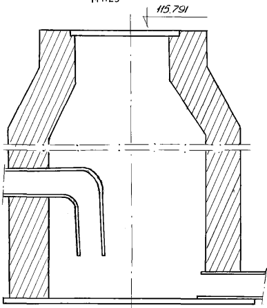
Чертеж колодца М 1:25
