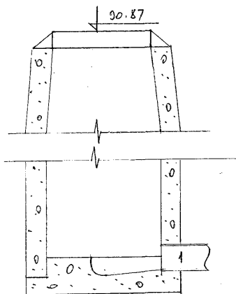
Чертеж колодца М 1:25
