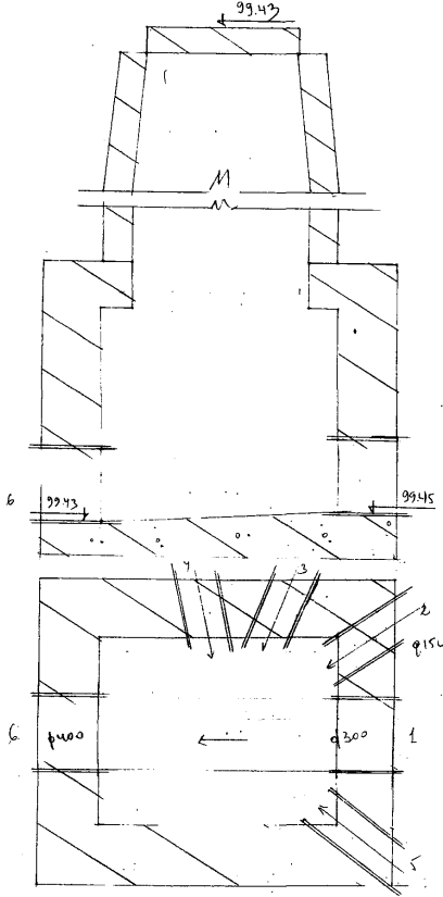
Чертеж колодца М 1:25
